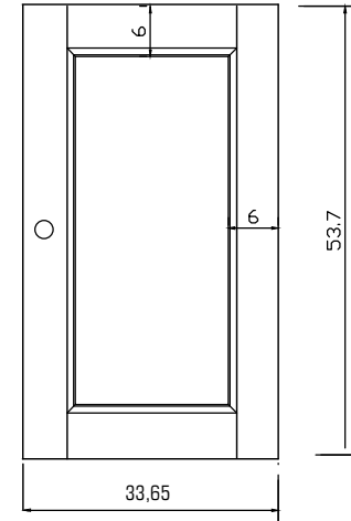
DETAIL DOOR
